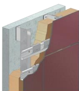
SISTEMA REMACHADO
