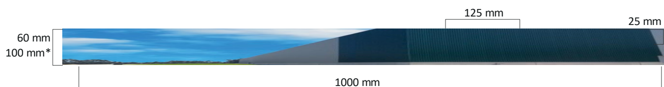
DETALLE JUNTA
