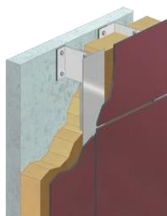
SISTEMA COLGADO
